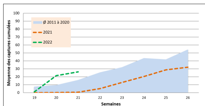
Figure 2 : Evolution des captures cumulées de la tordeuse du pois
