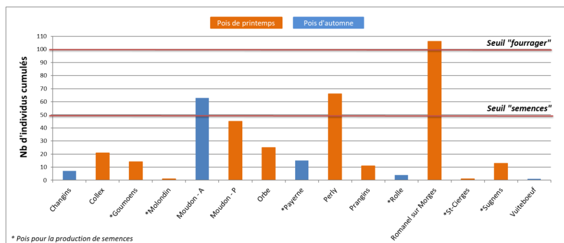
Figure 1 : Captures cumulées de la tordeuse du pois en 2022
